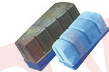
AT-08 菱苦土花岗岩磨料 Magnesia fickert briert brick for granite 规格 Specification: L140, L170 Grit: 8#, 16#, 24#, 36#, 46#, 60#, 80#, 120#, 220#, 240#, 320#, 400#, 600#, 800#, 1200#, 1500#
